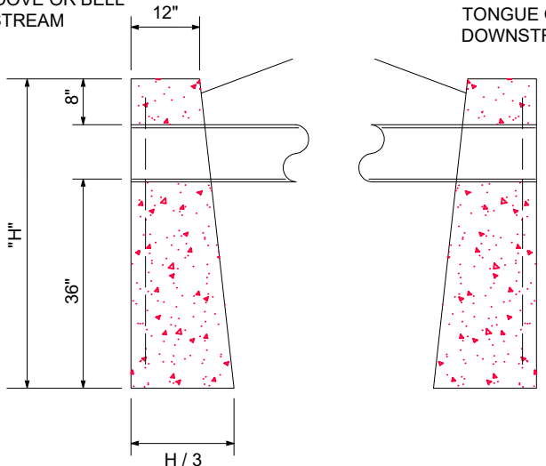
RIGID PIPE
