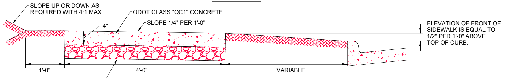
SECTION A-A
