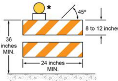
Type 2 Barricade
