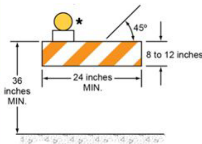
Type 1 Barricade
